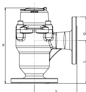
Abmessungen
