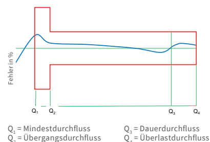
Typische Fehlerkurve
