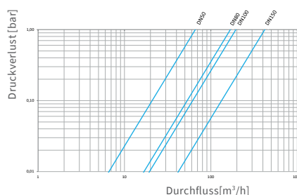
Druckverlustkurve
