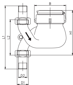
Abmessungen
