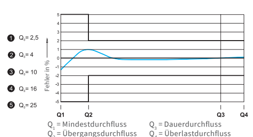
Typische Fehlerkurve
