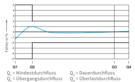
Typische Fehlerkurve
