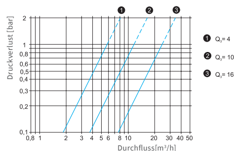
Typische Druckverlustkurve
