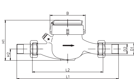
Abmessungen
