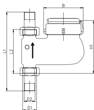
Abmessungen
